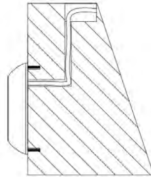
(4) Acabado / Finish
